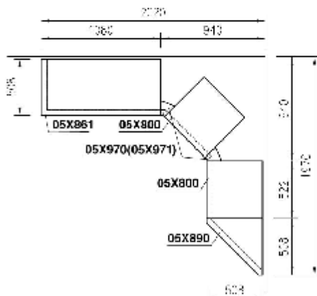
Půdorysná sestava 2
