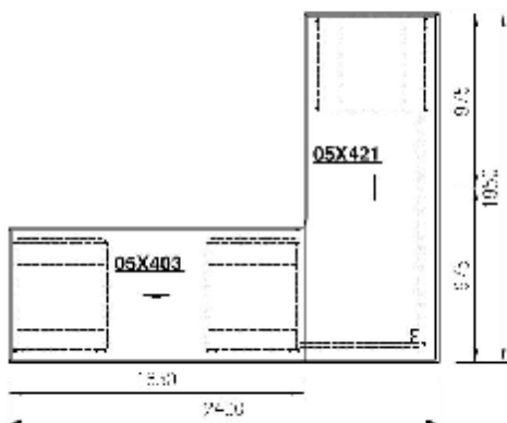
Prostorová sestava pravoúhlá—levá
