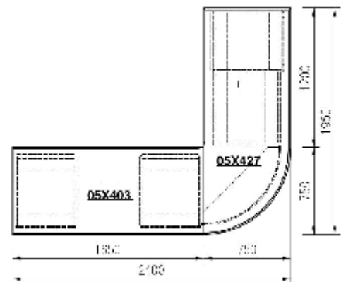
Půdorysná sestava s oblým rohem—levá (pravá)
