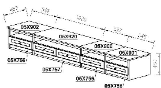
Prostorová sestava TV skříněk.
