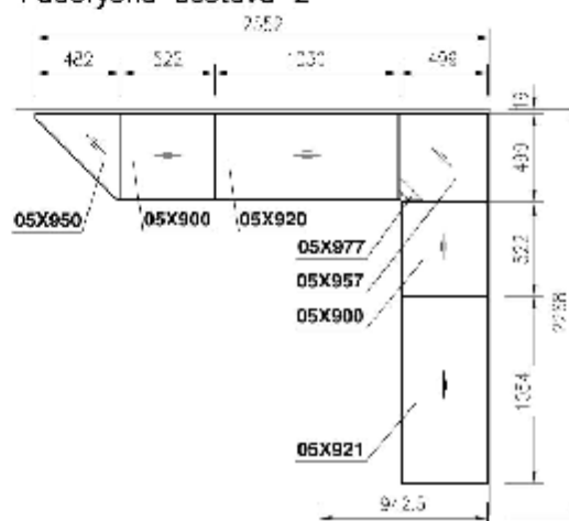
Půdorysná sestava 2
