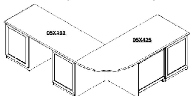
Prostor.sest. s oblým rohem otevřeným—levá.
