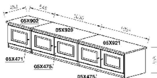
Prostorová sestava skříněk spodních.
