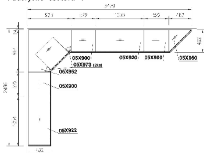
Půdorysná sestava 1
