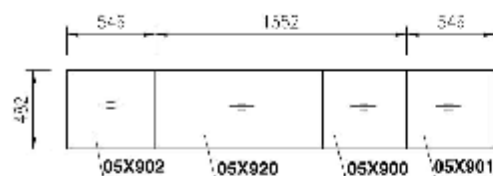
Půdorysná sestava TV skříněk.
