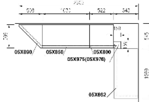
Půdorysná sestava 3
