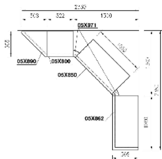
Půdorysná sestava 1
